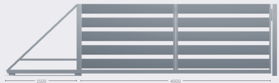
Brama przesuwna 200
